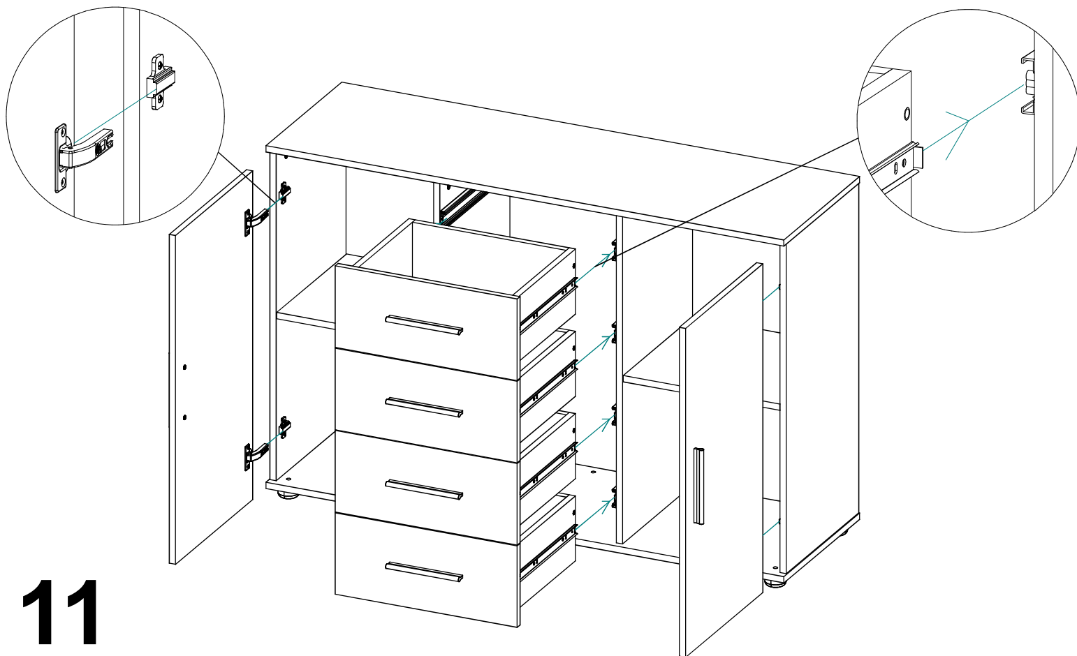
Загальний вигляд виробу
